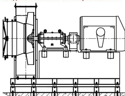
ИСПОЛНЕНИЕ 3 На едином постаменте и виброосновании
