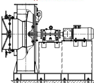
ИСПОЛНЕНИЕ 3 На едином постаменте
