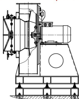
ИСПОЛНЕНИЕ 3 На едином постаменте и виброосновании
