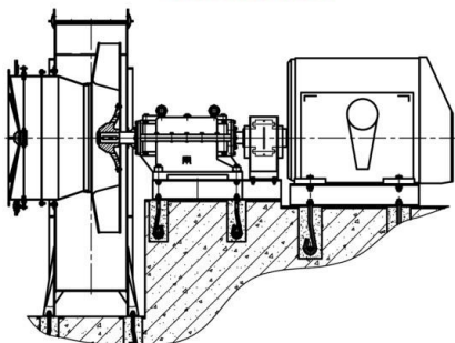
ИСПОЛНЕНИЕ 3 На едином постаменте
