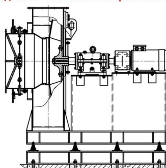
ИСПОЛНЕНИЕ 3 На едином постаменте и виброосновании
