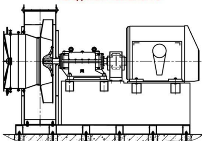
ИСПОЛНЕНИЕ 3 На едином постаменте
